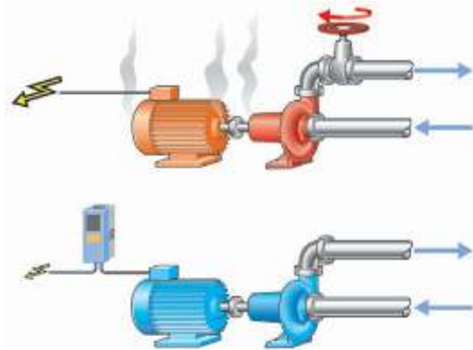
Рис. 1. Принцип энергосбережения при ПЧ-регулировании скорости вращения
