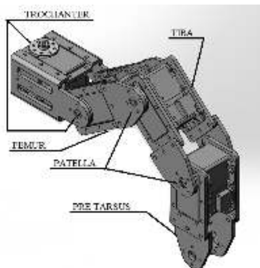
Рисунок 5. Внешний вид ноги. Датчик касания (лапка и коготки) отсутствуют
