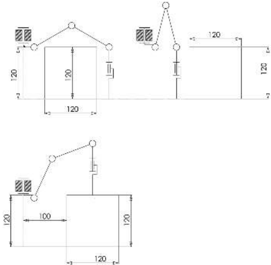
Рисунок 2. Опорные точки преодоления препятствия
