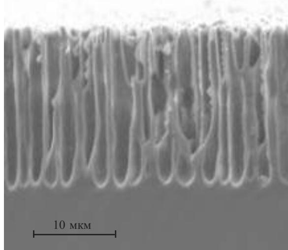
Рис. 2. Колоннообразная текстура пористого кремния на шлифе приповерхностной зоны фронтальной поверхности кремниевой подложки
