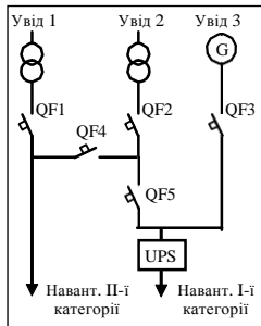
Рис. 11. Система АВР з трьома вводами, один з яких є автономним генератором, секціонуванням, навантагами I та II категорій та джерелом безперебійного живлення
