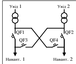
Рис. 10. Система АВР з двома вводами та двома секціями живлення навантаг
