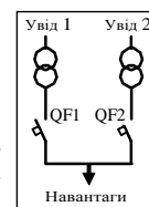
Рис. 2. Система АВР з двома трансформаторними уводами та спільною секцією живлення наванта
