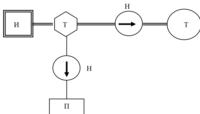
Рис. 1 – Простая схема использования теплоты: И – источник теплоты; Т – теплообменный аппарат; П – потребитель теплоты; Н – нагнетатель; Тр – дымовая труба
