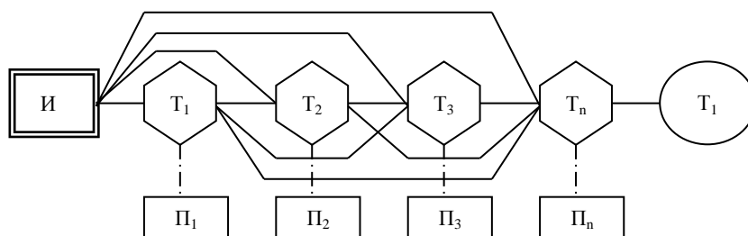
Рис. 2 – Обобщенная схема использования теплоты
