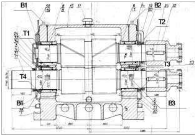
Рис. 3. Точки измерения вибрации и температуры на шестеренной клетке: B1, B2, B3, B4 – датчики вибрации; T1, T2, T3, T4 – датчики температуры
