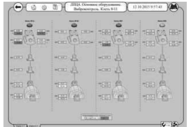
Рис. 5. Мнемосхема вибрационного состояния чистовой группы клетей 8-11
