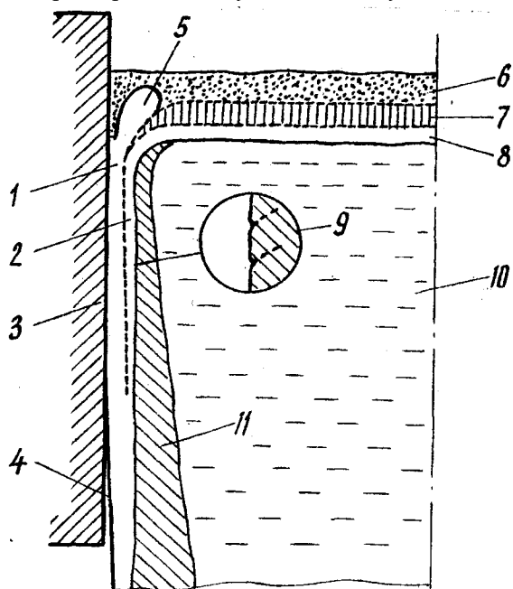
Рис.1 - Схематическое изображение состояния слоев ШОС в кристаллизаторе МНЛЗ
