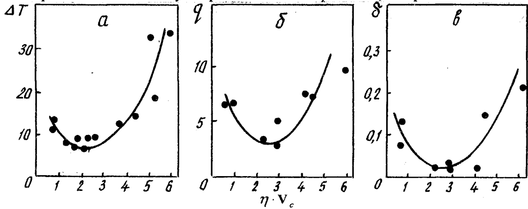
Рис.2 - Зависимость между произведением \eta \cdot V_c (пуаз · м /мин) и (а) изменением температуры в кристаллизаторе, \Delta T (° С/мин), (б) тепловым потоком в кристаллизаторе, q (Mкал/м 2 ·ч) и (в) толщиной жидкой пленки шлака, \delta (мм).
