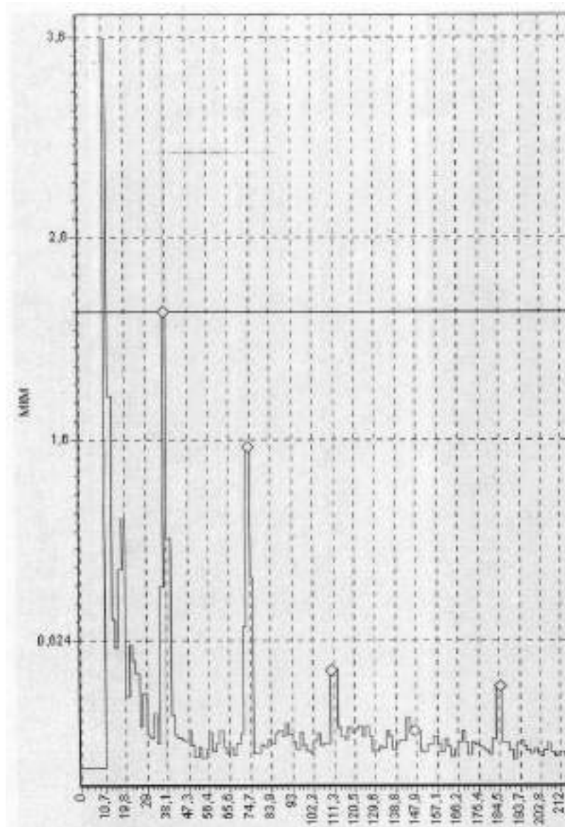
Рис. 3. Фрагмент записи вибраций шпинделя шлифовального круга
