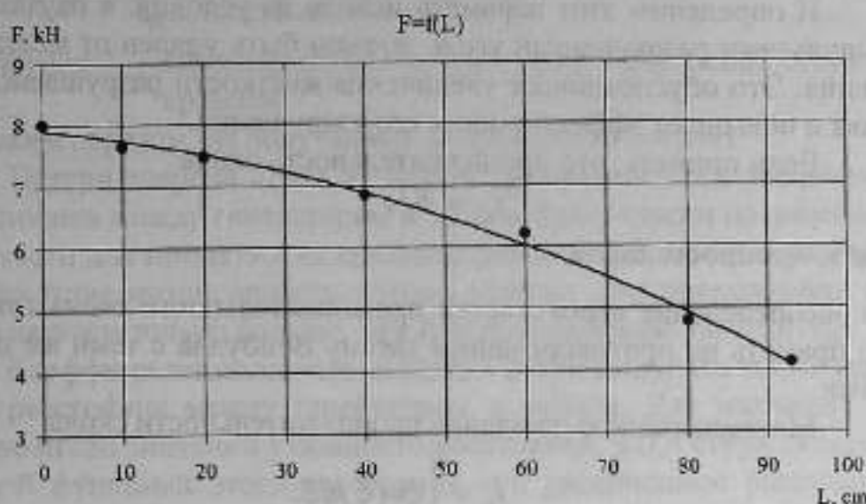
Рисунок 2 – Зависимость силы удара гидроимпульсной струи от толщины угольного слоя для насадка диаметром 12мм.
