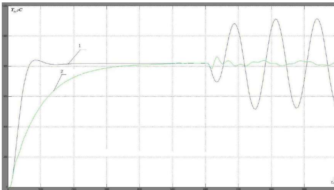
Рис. 2. Результаты сравнительного моделирования традиционной и предложенной двухконтурной системы управления топки НТКС (1 –моделирование системы по контуру «Топливо»; 2 - моделирование системы с коррекцией по воздуху)
