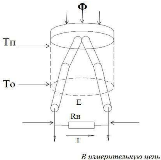
Рисунок 1 – Конструкция ТЭП
