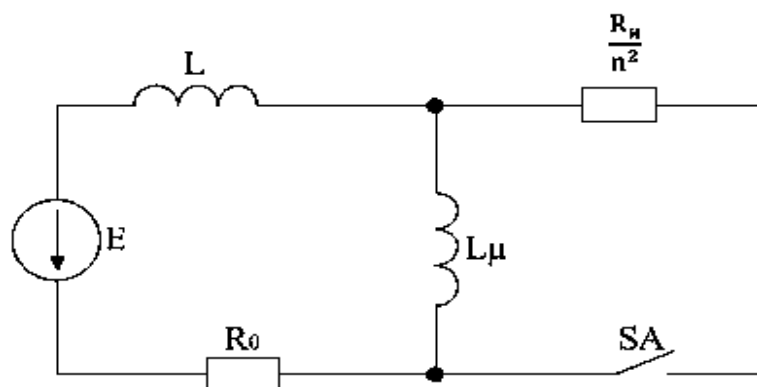
Рисунок 2 – Эквивалентная схема устройства, приведенная к первичной обмотки трансформатора
