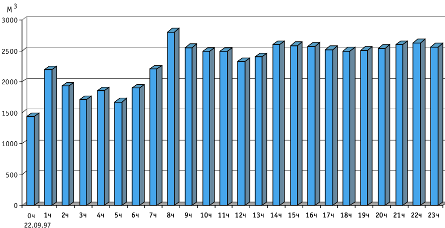
Рис. 8. Суточная расходограмма
