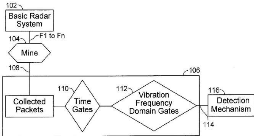
Рис.1. Структурна схема датчика радара
