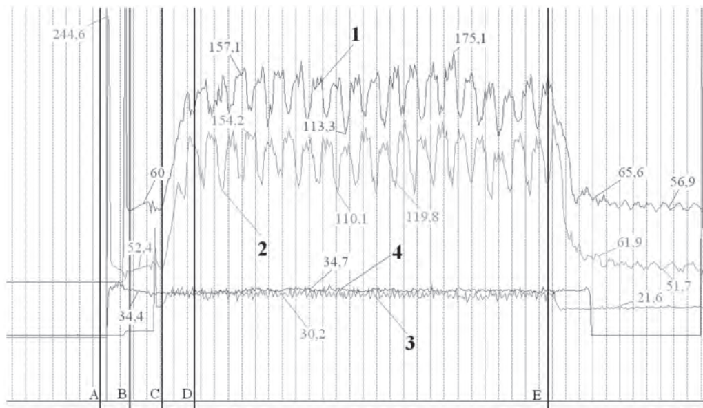
Рис. 1. Изменение мгновенных значений потребляемой активной мощности электродвигателей: 1, 2 – приводы относительного движения резовых дисков; 3 – привод отбойного устройства; 4 – привод конвейера. Шаг линий сетки – 5 с (сносками обозначены мгновенные значения активных мощностей)
