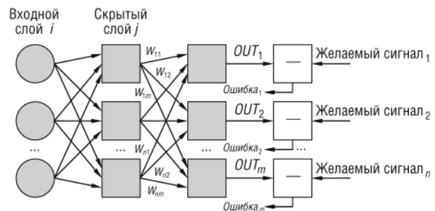
Рис.1. Обобщенная структура двухслойной нейронной сети для реализации алгоритма обратного распространения ошибки
