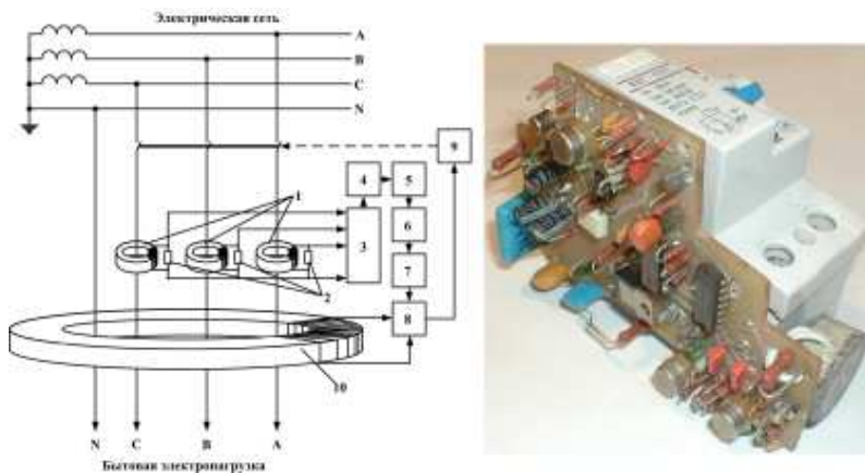
Рис.4 – Защита, реагирующая на искрение ослабленного силового контактного соединения в электрической сети, встроенная в серийно выпускаемое УЗО
