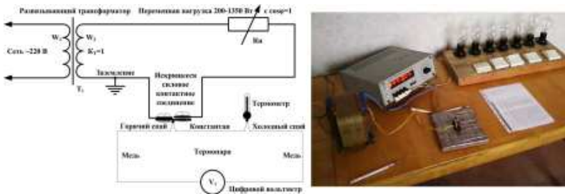
Рис.1 – Схема и стенд для измерения температуры искрящегося силового контактного соединения
