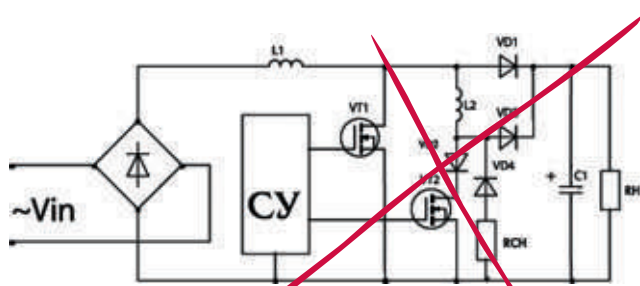
Традиционное решение с ZVS на базе контроллера UC 3855 (Unitrode)
