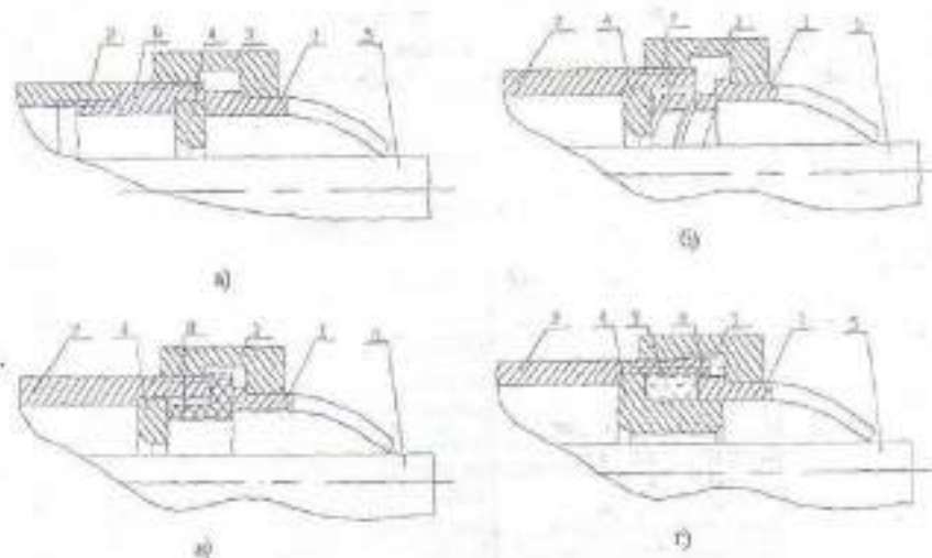
Рисунок 1 - Варианты сборного подающего патрона с различными связями упругой рабочей части с зубчатой передачей: а - жесткой; б - упругой; в - демпфирующей; г - упруго-демпфирующей
