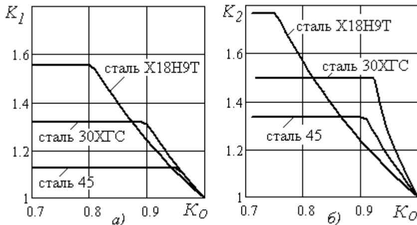
Рис. 2. Графіки зміни коефіцієнтів підвищення продуктивності K від коефіцієнта зниження температури K_O для різних сталей під час чорнкової обробки – а) та чистової обробки - б)
