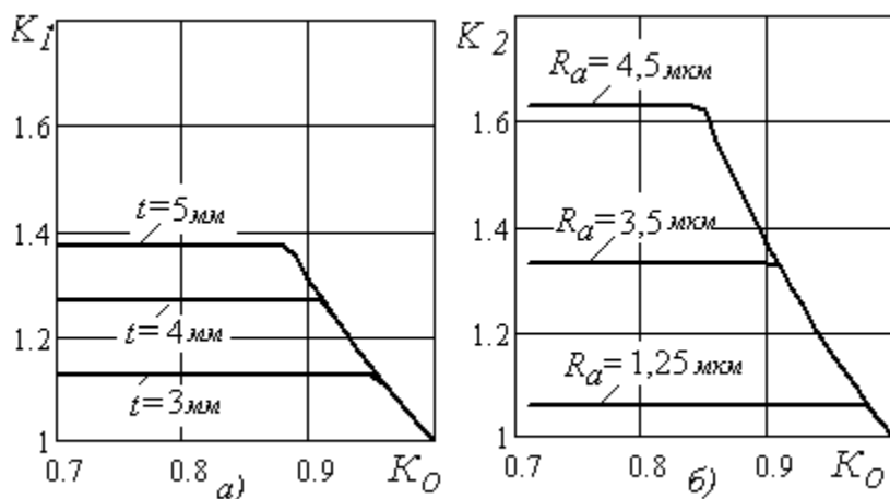
Рис. 4. Графіки зміни коефіцієнтів підвищення продуктивності K_{II} від коефіцієнта зниження температури K_O для різних глибин різання t та шорсткостей поверхні R_a під час чорнкової обробки а) та чистової обробки - б)
