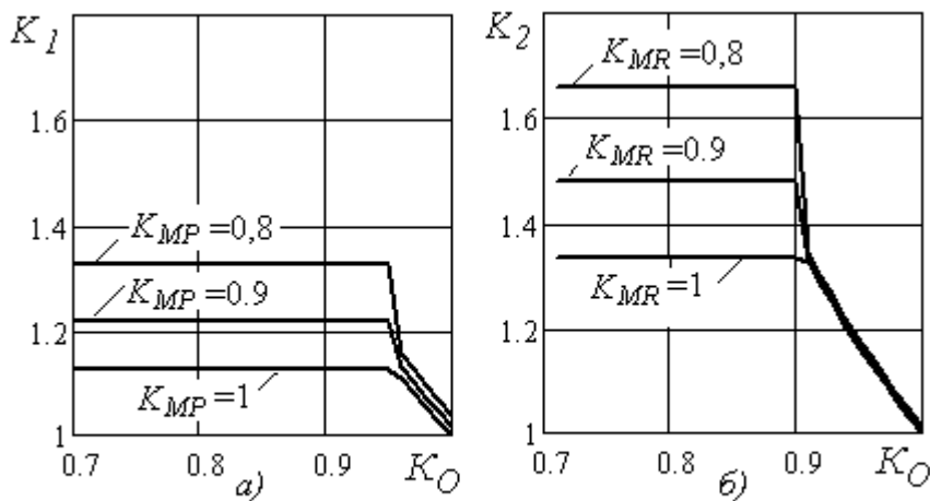
Рис. 3. Графіки зміни коефіцієнтів підвищення продуктивності K_{II} від коефіцієнта зниження температури K_O для різних коефіцієнтів K_{MP} та K_{MR} , що враховують мастильну дію МОТС, під час чорнкової обробки – а) та чистової обробки - б)
