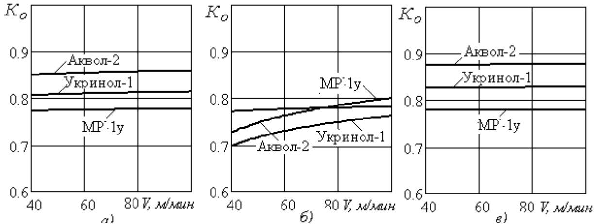
Рис. 5. Графіки залежності коефіцієнта зниження температури різання K_o від швидкості V під час обробки сталі 45 з подачею МОТС вільним поливом - а) напірним струменем - б) та розпиленням - в)
