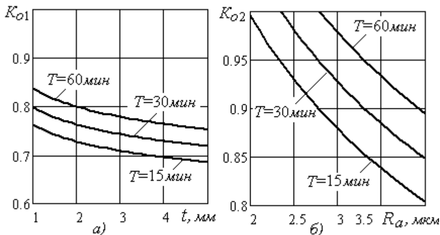
Рис. 1. Графіки зміни граничних коефіцієнтів K_{O1} та K_{O2} від глибини різання t під час чорнової обробки – а) та шорсткості обробленої поверхні R_a під час чистової обробки – б)
