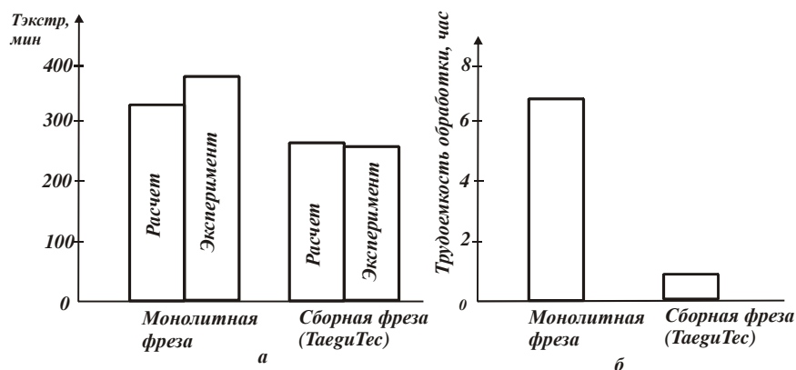
Рисунок 2 – Диаграммы распределения параметров T_{экспр} (а) и трудоемкости обработки (б) монолитной и сборной концевыми фрезами.
