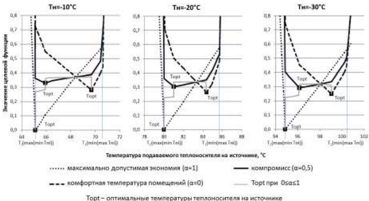
Рис. 3. Значения целевой функции при различных весах \alpha
