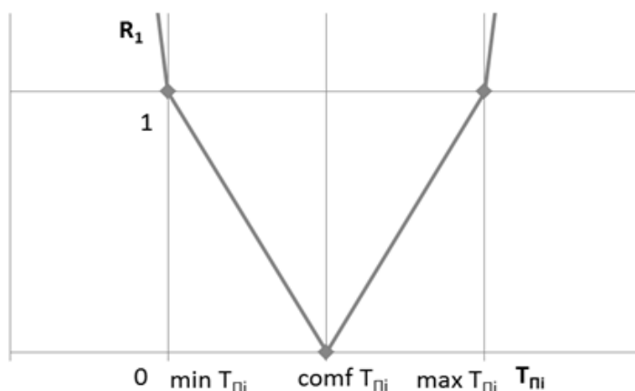
Рис. 1. График штрафной функции температуры воздуха в помещениях
