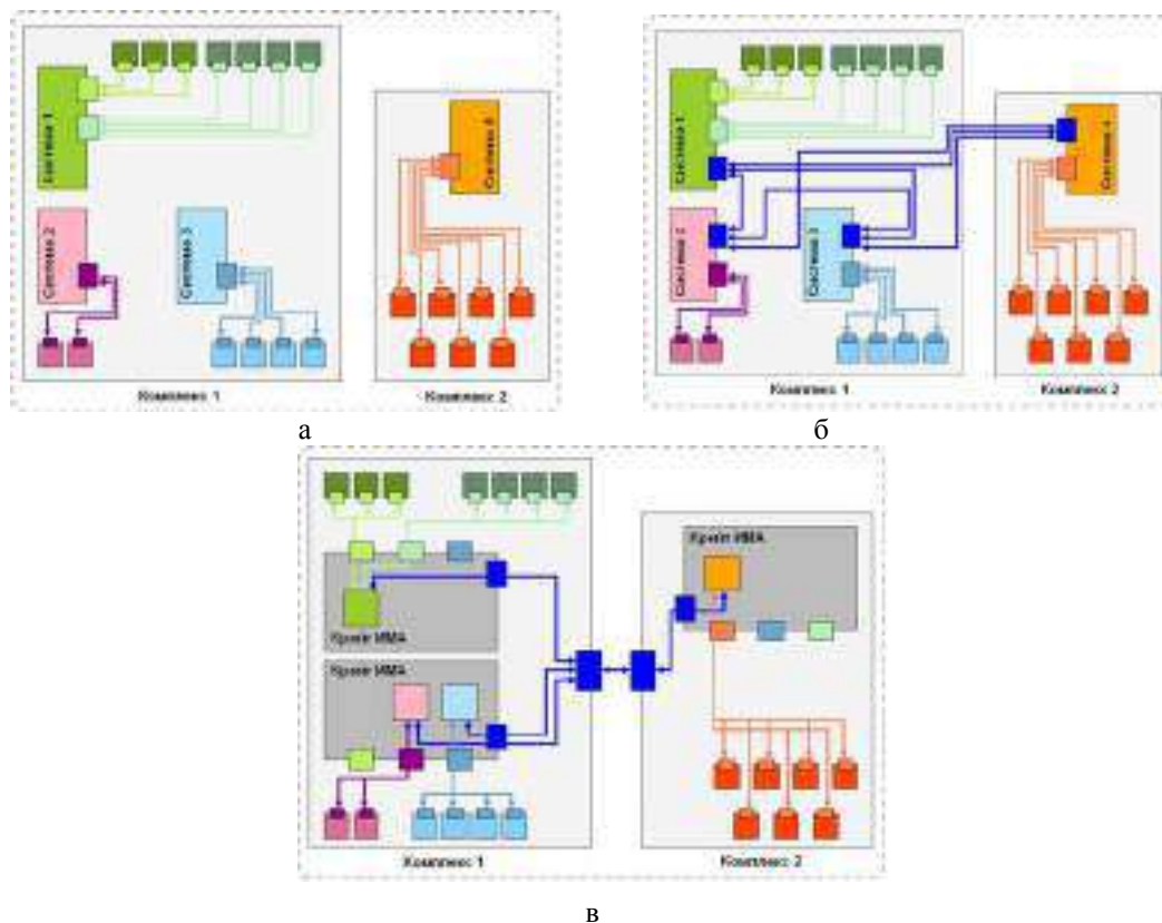
Рис. 4. Примеры построения структур авиационных комплексов: независимый принцип построения архитектуры БРЭО (а); федеративный принцип построения архитектуры БРЭО (б); интегрированный модульный принцип построения архитектуры БРЭО (в) (ИМА – интегрированная модульная авионика)
