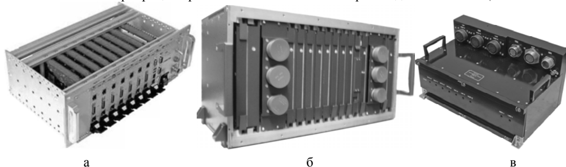
Рис. 1. Бортвые цифровые вычислительные системы структуры ИМА: разработки ЗАО НПФ «Авиационная и Морская Электроника» (а); разработки ФГУП «СПб ОКБ «Электроавтоматика» им. П. А. Ефимова» (б); разработки ОАО «РПКБ «Раменское» (в) (примеры)
