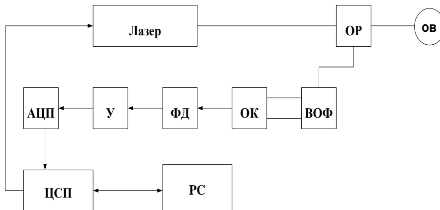
Рис. 3 - Схема системы контроля на основе рамановского излучения
