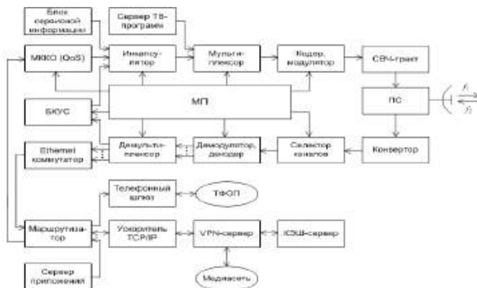
Рисунок 1 – Структурная схема центральной станции сопряжения
