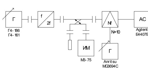
Рисунок 2 – Схема измерения характеристик смесителя на гармониках
