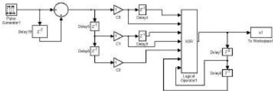
Рис. 1 – Структурная схема кодирующего устройства (7,3)
