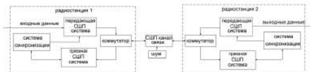
Рис.2 – Обобщенная структурная схема СШП системы связи с повышенной точностью и стабильностью синхронизации
