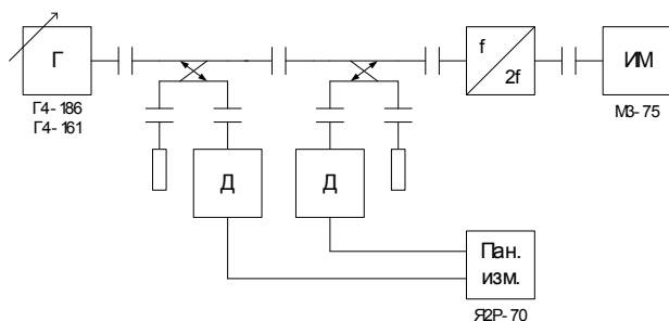
Рисунок 1 – Схема измерения характеристик умножителей частоты
