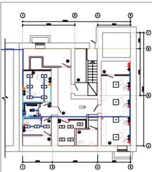
Рис. 9. План расположения оборудования с подсвеченной трассой прокладки кабеля от группы ЩР
