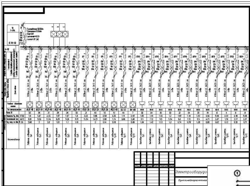
Рис. 3. Однолинейная схема
