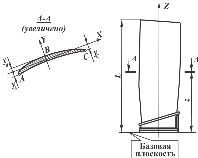
Рис. 1. Лопатка 3-й ступени компрессора ГТД ТВ3-117
