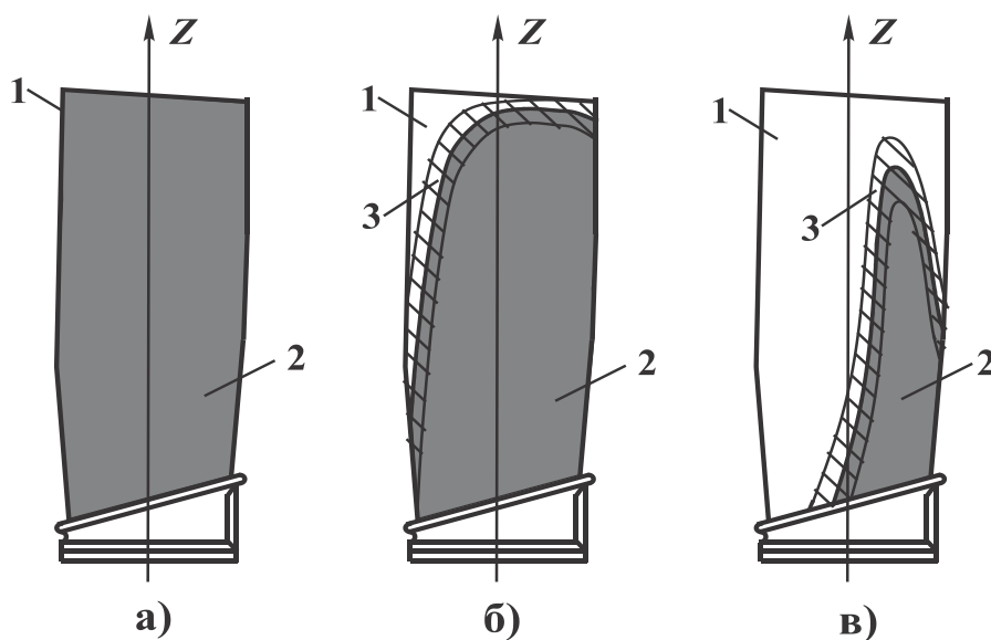
Рис. 2. Особенности разрушения ионно-плазменного покрытия лопатки:
