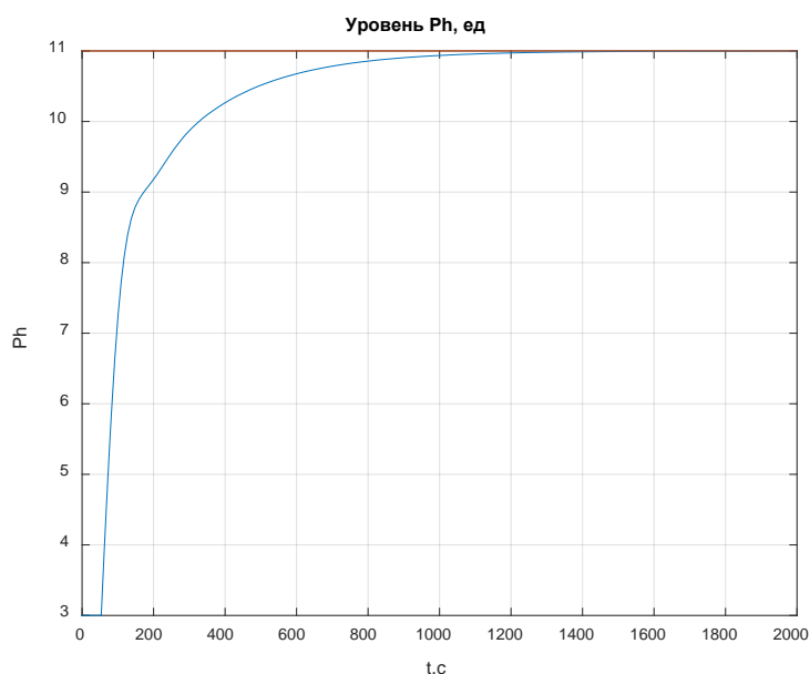
Рисунок 4 – График переходного процесса уровня рН
