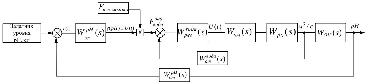
Рисунок 1 – Структурная схема САР уровнем рН
