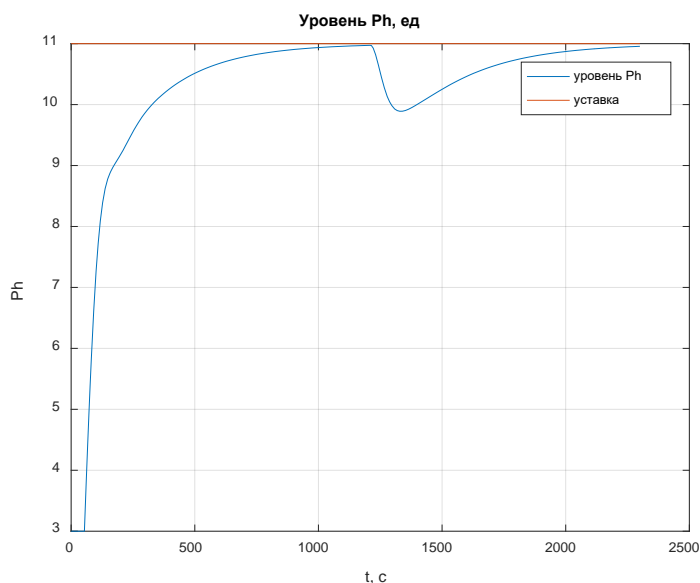
Рисунок 5 – Переходной процесс уровня рН при изменении расхода известкового молока с 40 \text{ м}^3/\text{с} до 35 \text{ м}^3/\text{с}
