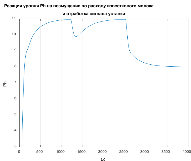
Рисунок 8 – Переходной процесс рН при изменении сигнала уставки
