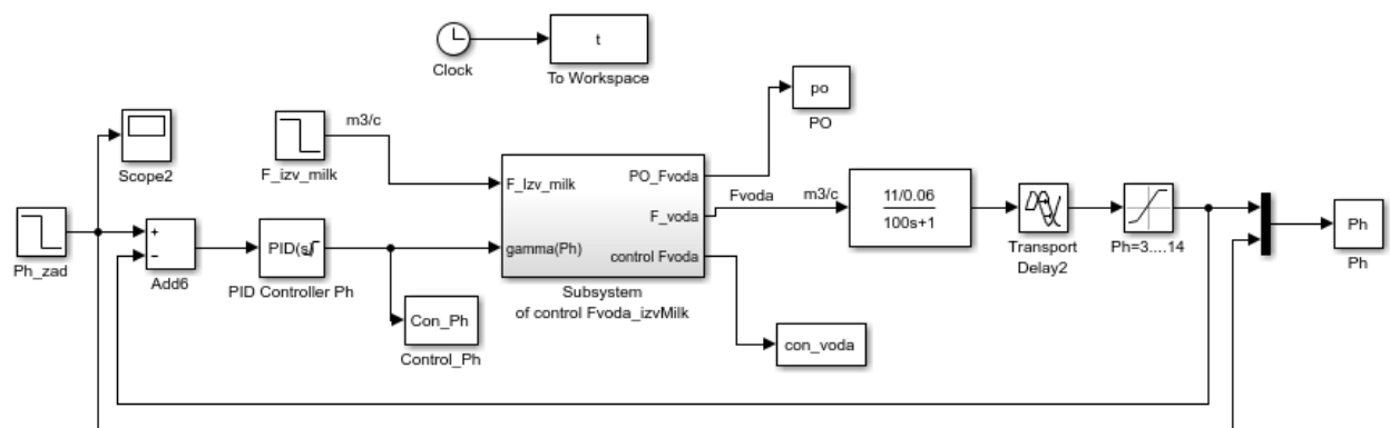
Рисунок 3 – Схема моделирования каскадной двухконтурной САР уровня рН
