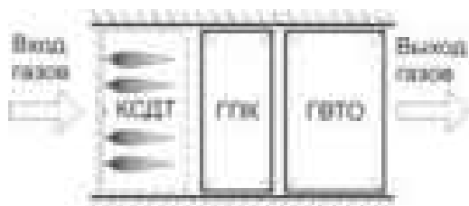
Рис. 2. Фрагмент газового тракта КУ (вариант 2)
