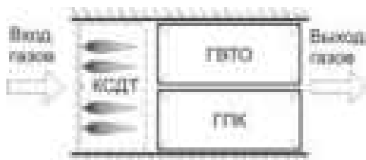
Рис. 3. Фрагмент газового тракта КУ (вариант 3)
