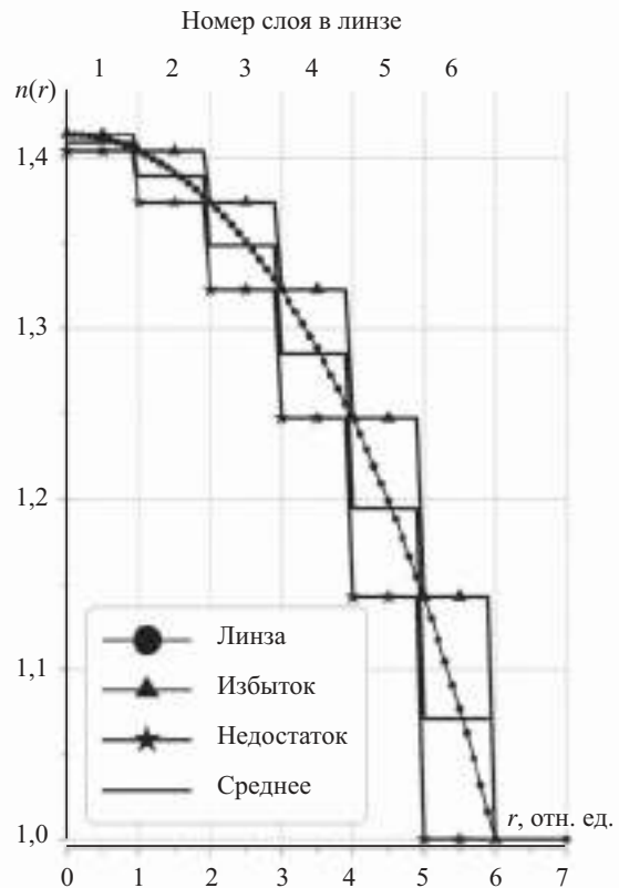
Рис. 2. Модельные зависимости показателя преломления линзы Люнеберга от расстояния до ее оси
