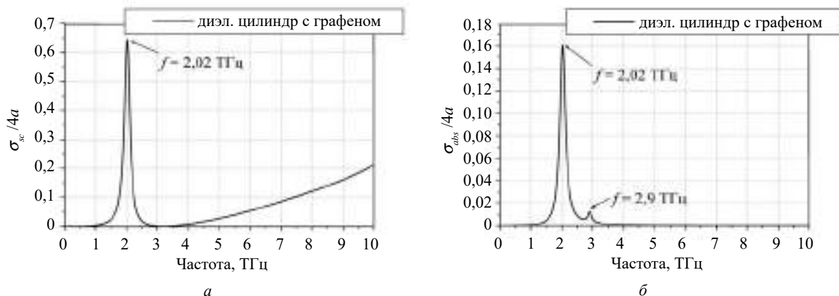
Рис. 6. Графики зависимости нормированных сечений рассеяния ( а ) и поглощения ( б ) от частоты для диэлектрического цилиндра радиусом a = 6 мкм с графеновым покрытием ( n = 1,5 )
