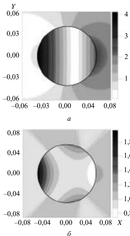
Рис. 7. Пространственное распределение компоненты поля |H_z| для диэлектрического цилиндра со слоем графена на частотах падающего излучения f = 2,02 ТГц (а) и f = 2,9 ТГц (б)
