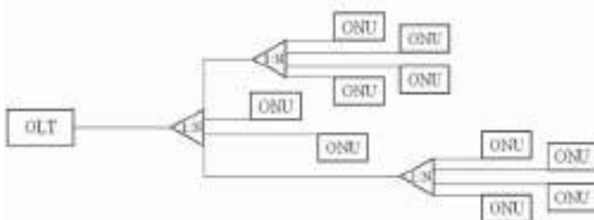
Рис. 6. Топология «Дерево»
