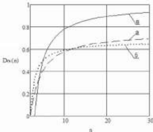
Рис. 5. Зависимости живучести сетей от их размера при разрыве одной дуги: а – шпинная PON; б – линейная сеть; в – звездообразная сеть PON
