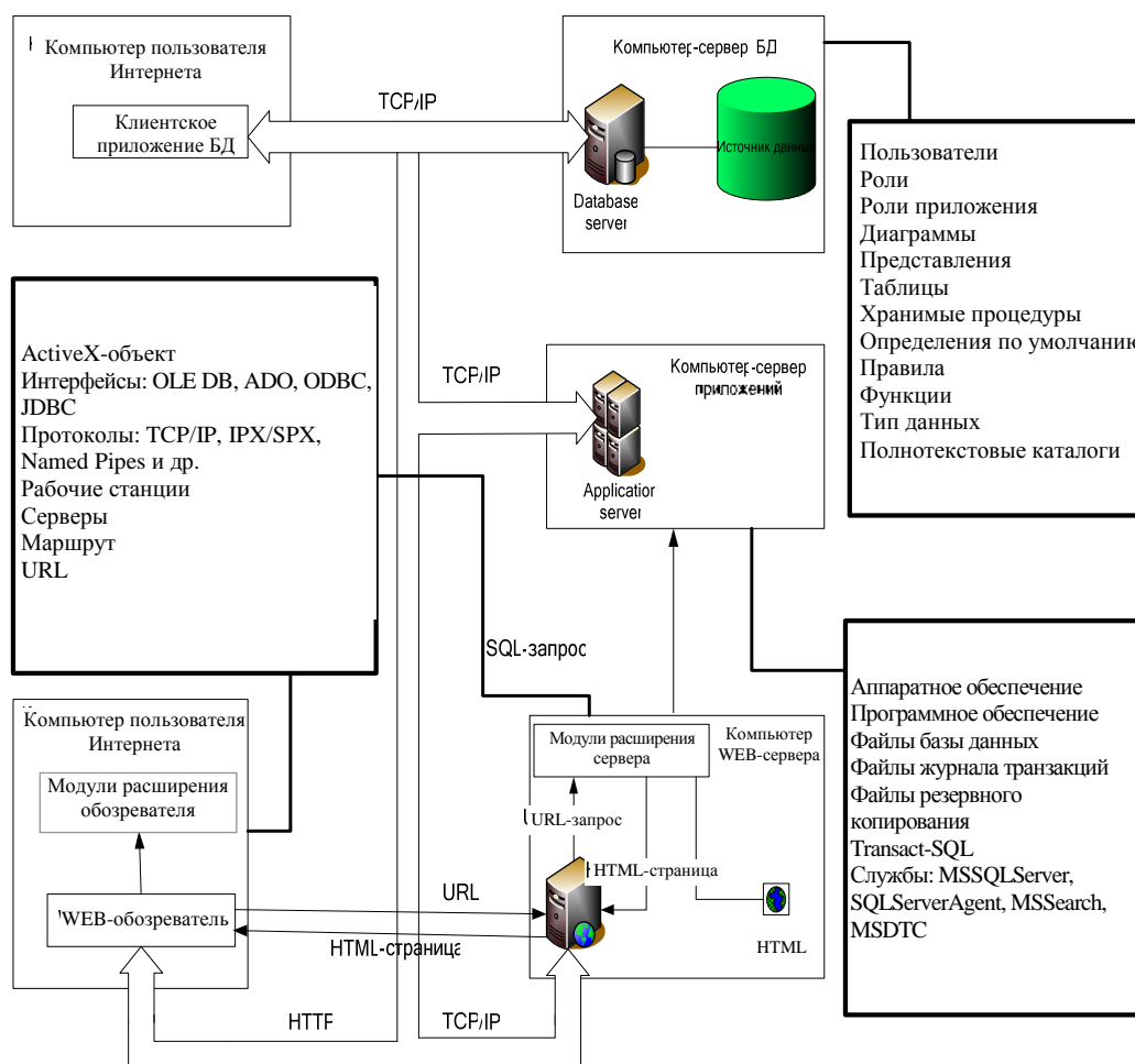
Объекты воздействия на фоне многоуровневой архитектуры СУБД
