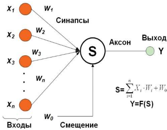
Рис. 4. Структура искусственного нейрона
