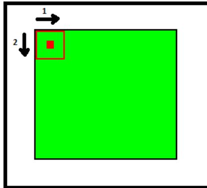
Рисунок 2 – Операция valid-свертки [3]
