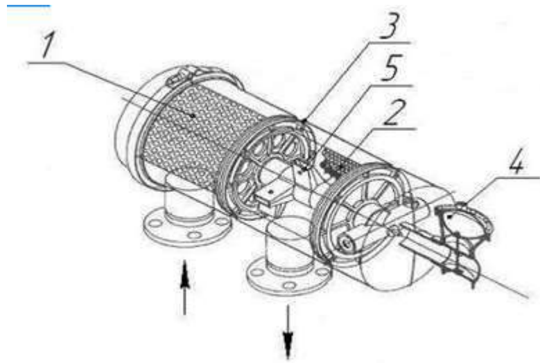
Рисунок 1 – Конструкція фільтра Tekleen серій OBF
