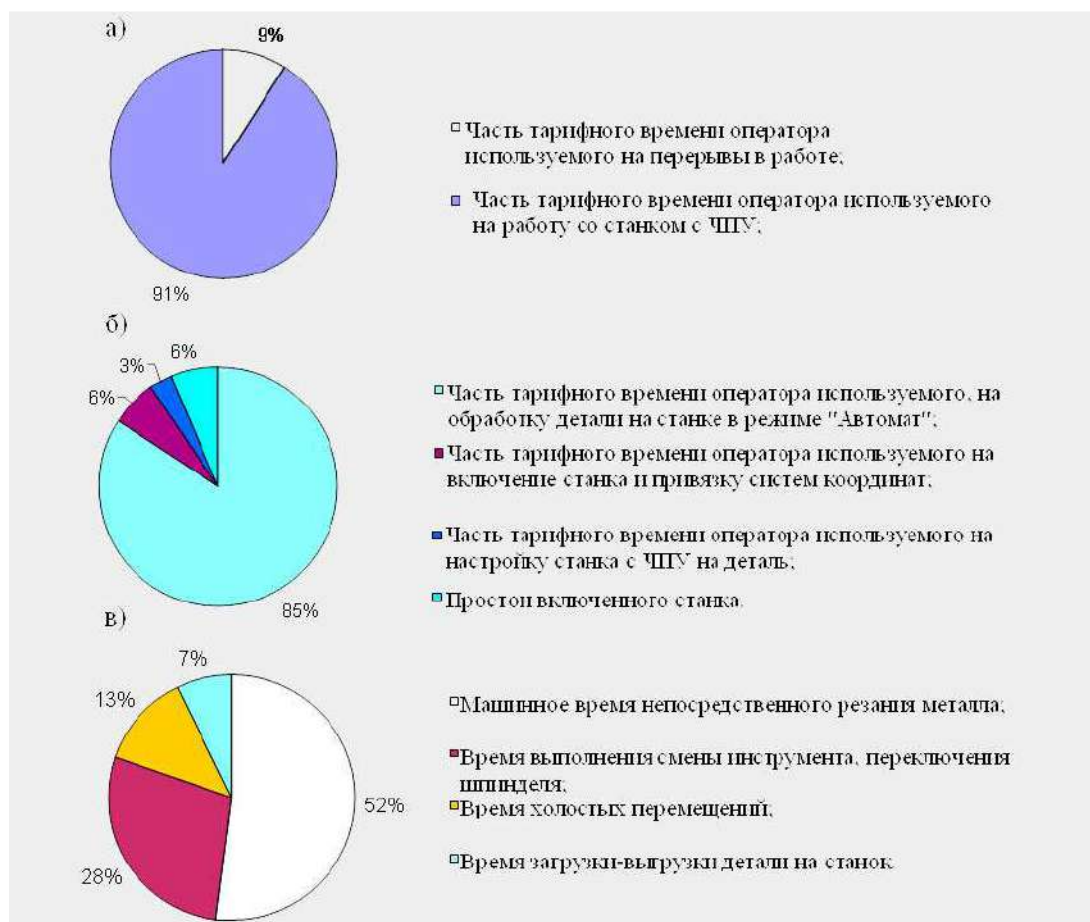
Рис. 1. Диаграммы оценки потраченного времени в ходе обработки корпусной детали на токарно-револьверном станке с ЧПУ Haas SF20
