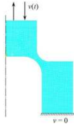
Рис. 4. Конечно-элементная сетка в осевом сечении образца типа «колокольчик»
