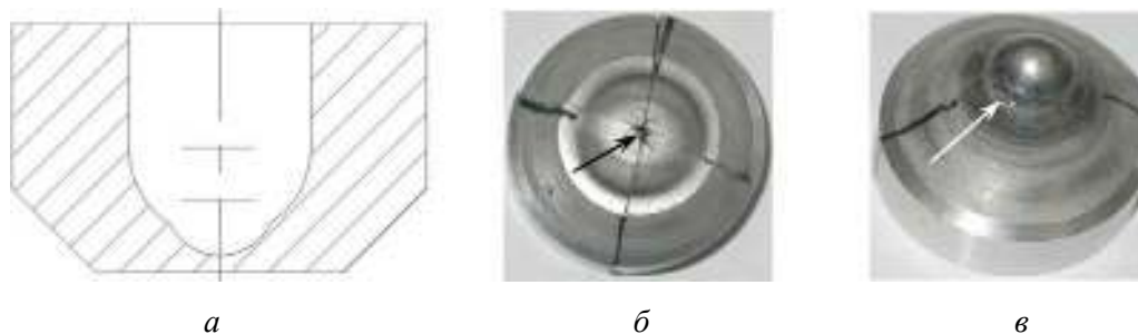
Рис. 7. Образец в виде толстостенного стаканчика с утонением на доньшке: a – продольное сечение в исходном состоянии (эскиз); фото образцов после испытаний без подпора доньшка ( б ) и с подпором ( в ). Стрелками указаны места первоначального разрушения
