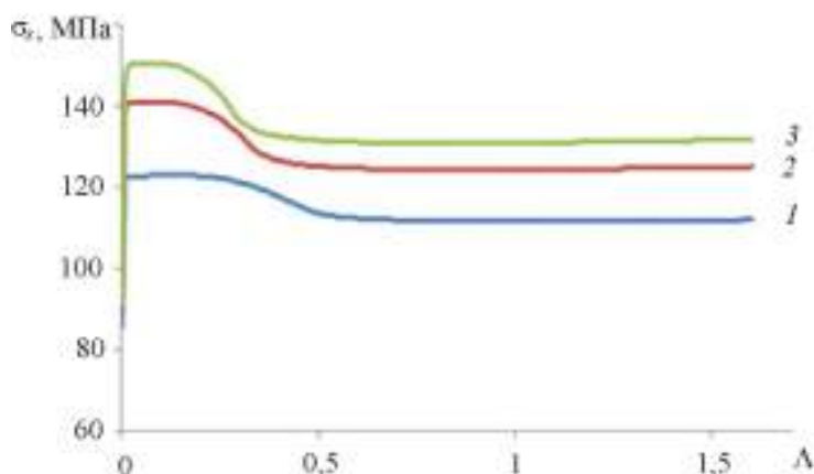
Рис. 2. Зависимость сопротивления деформации \sigma_s от степени деформации сдвига \Lambda при скорости деформации сдвига H : 1 – 0,1; 2 – 0,3; 3 – 0,5 \text{c}^{-1}
