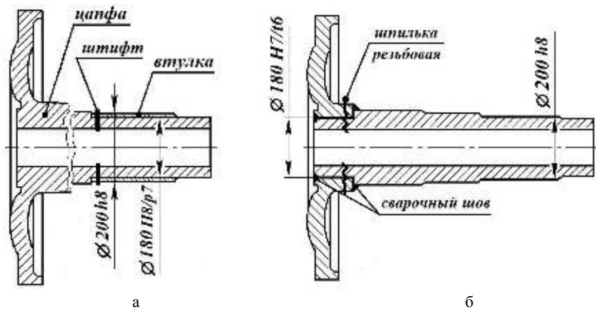
а – с установкой ремонтной втулки; б – запрессовкой новой стержневой части с сохранением крышки
