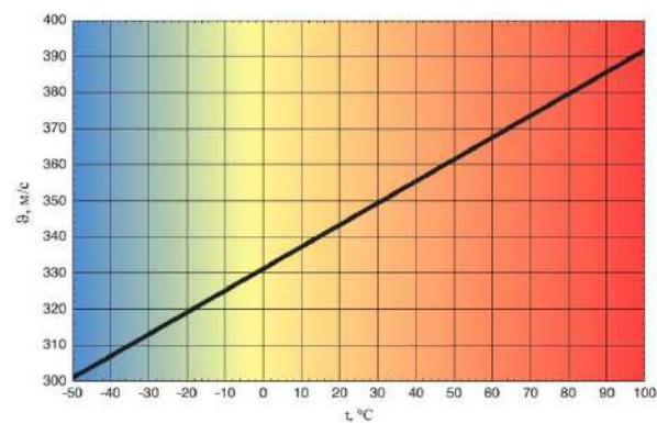
Рис. 5 Зависимость скорости звука от температуры
