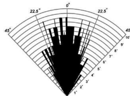
Рис. 3. Диаграмма направленности ультразвуковой волны
