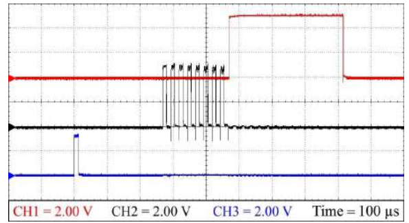
Рис. 11. Вид трёх сигналов снятых с входа «Trig» (синий), с модуля при генерации звукового сигнала (чёрный) и с выхода «Echo» (красный)
