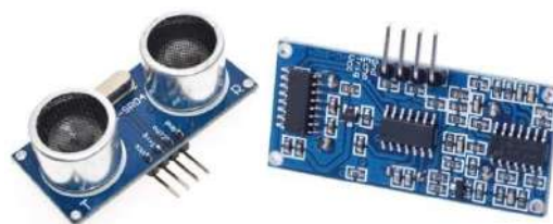
Рис. 1. Ультразвуковой дальномер HC-SR04
