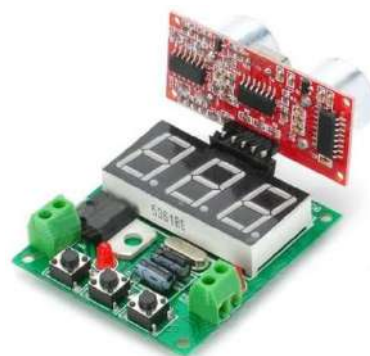
Рис. 16. Модуль DYP-ME008 и ультразвуковой дальномер DYP-ME007
