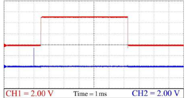
Рис. 10. Сигнал на выходе «Echo» с длительностью пропорциональной расстоянию в 100 см (красный) и сигнал на входе «Trig» (синий)
