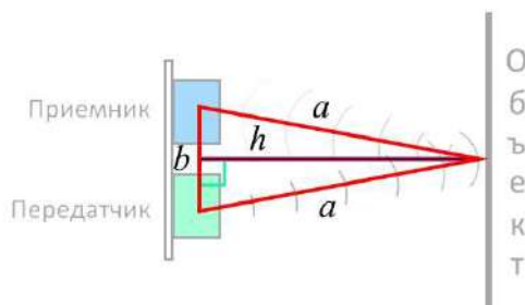
Рис. 6. Геометрическое представление распространения звуковой волны
