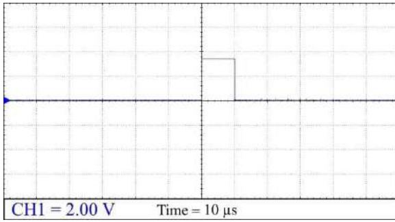
Рис. 8. Сигнал, подаваемый микроконтроллером на вход «Trig»
