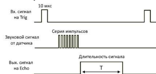
Рис. 7. Временная диаграмма сигналов дальномера
