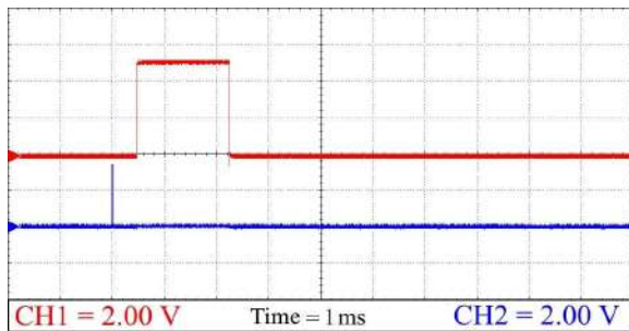
Рис. 9. Сигнал на выходе «Echo» с длительностью пропорциональной расстоянию в 30 см (красный) и сигнал на входе «Trig» (синий)
