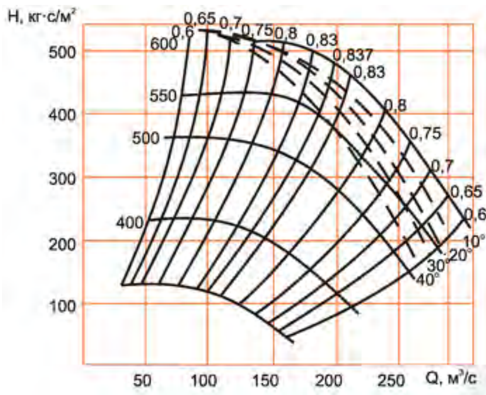
Рисунок 4 – Аэродинамические характеристики ВЦД-32
