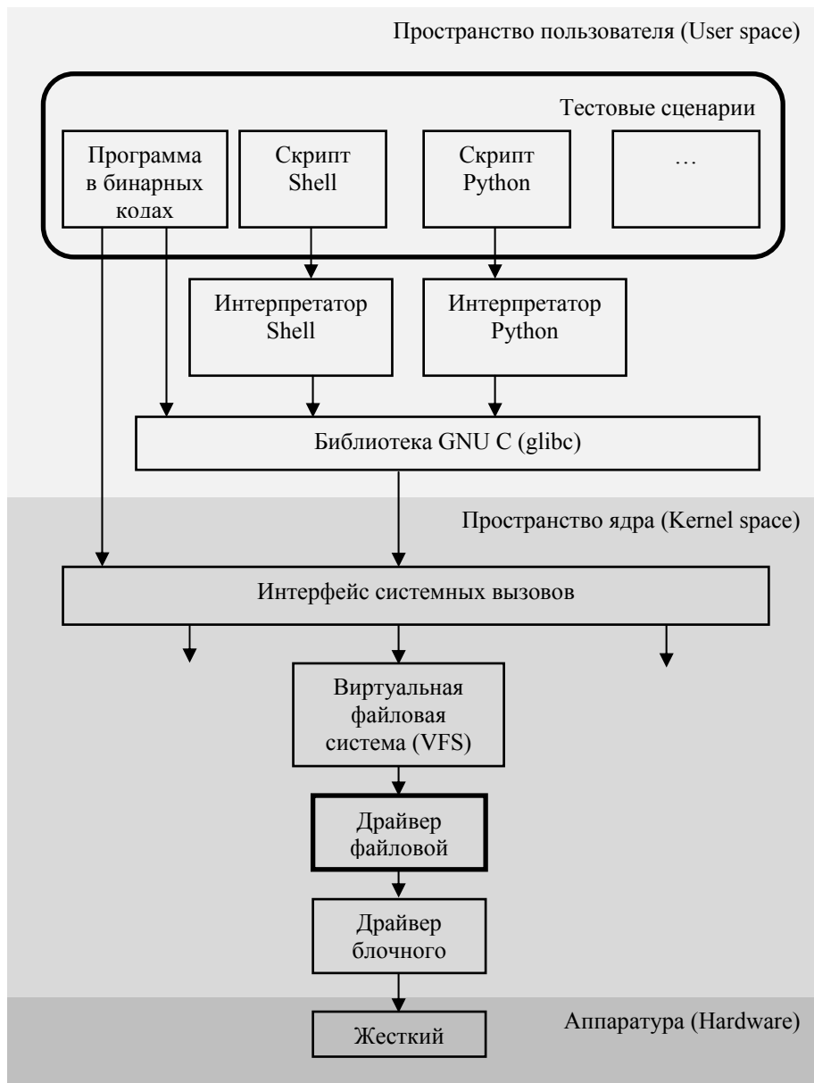
Рис. 1. Схема тестирования драйверов файловых систем.
