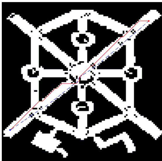
Рис. 2. Сравнение пути A^* (красная линия) с путем \Theta^* (синяя линия)
