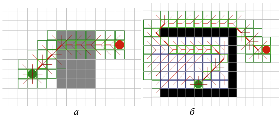
Рис. 1. Иллюстрация работы алгоритма «Лучший — Первый»: зеленый маркер — начало пути; красный маркер — конец пути; зеленый контур — анализируемые ячейки; красные линии — труднопроходимая зона; черные ячейки — непроходимая зона.
