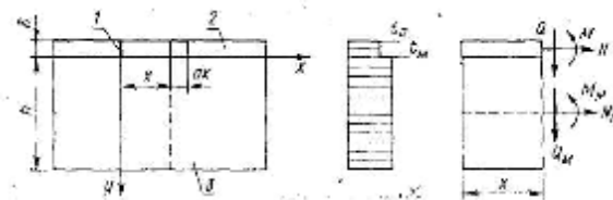
1 - трещина; 2 - окалины; 3 - металл
