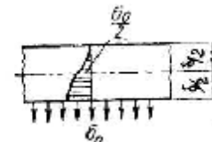
Рисунок 4 – Распределение нормальных напряжений по высоте окалины [7]
