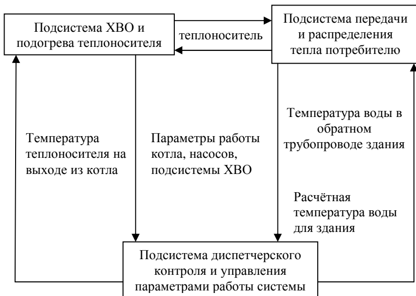
Рисунок 2 – Структура многоуровневой системы управления теплоснабжением
