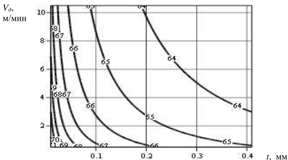
Рис. 1. Зависимость средней прочности m(\sigma_{po}) , МПа ситалла АС-418 в зависимости от скорости заготовки V_d , (м/мин) и глубины t (мм) резания при продольном круглом шлифовании кругом 1А1 200-10-3-60-76 АС6 125/100-4- М2-01 при V_k=30 м/с не превышает 0,4 %.
