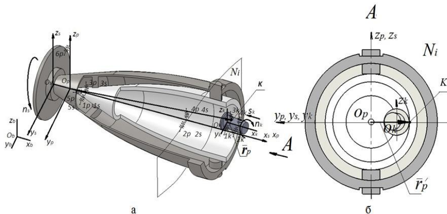
Рис. 1. Схема шлифования внутреннего профиля оболочки: а) расположение систем координат элементов технологической системы; б) проекция радиус-вектора \bar{r}_p точки поверхности детали в плоскости N_i ( \bar{r}_p )
