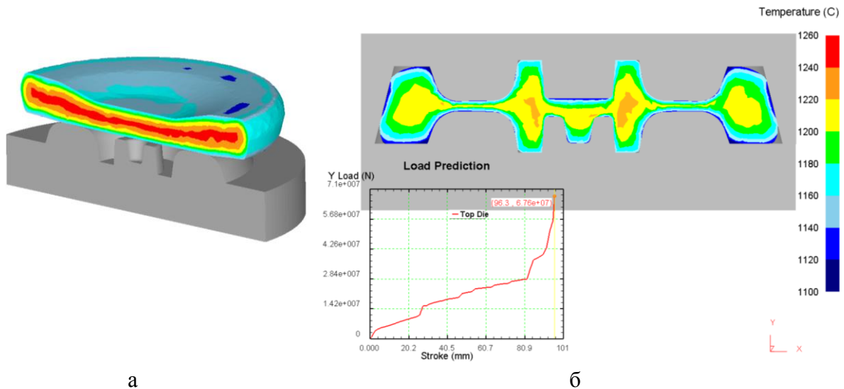
Рис. 6 – Заготовка после транспортировки, выдержки на нижнем штампе (а) и формовки (б) на прессе силой 100МН.
