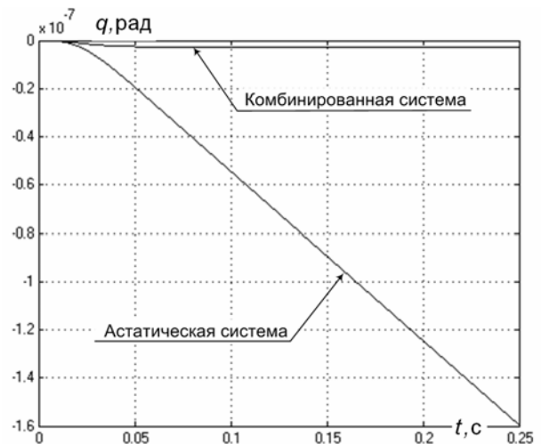
Рис. 10. Параболическая нагрузка
