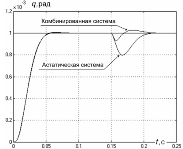
Рис. 8. Переходные процессы в астатической и комбинированной системах
