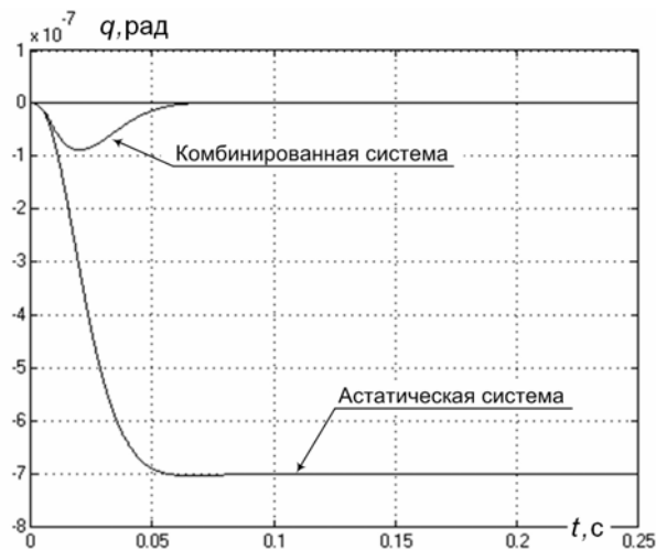
Рис. 9. Линейно нарастающая нагрузка
