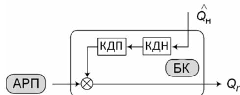
Рис. 7. Структурная схема блока компенсации
