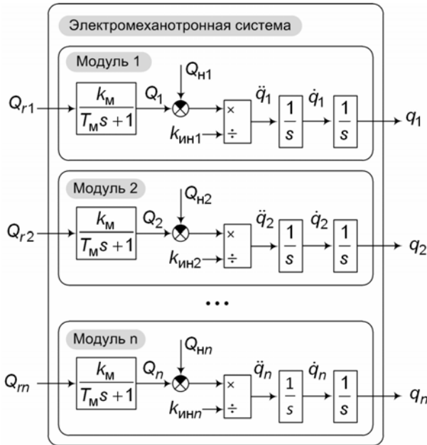
Рис. 1. Обобщенная структурная схема электромеханотронной системы
