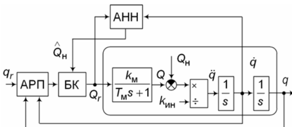
Рис. 2. Комбинированная система с компенсацией нагрузки
