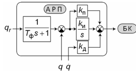
Рис. 3. Астатический регулятор положения
