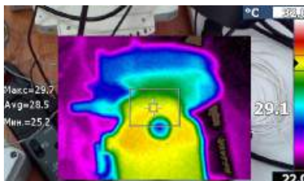
Рисунок 2. Термограмма подшипника электродвигателя
