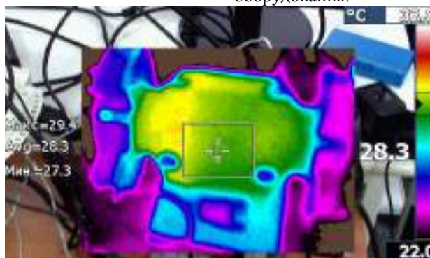
Рисунок 1. Общая термограмма диагностируемого электродвигателя
