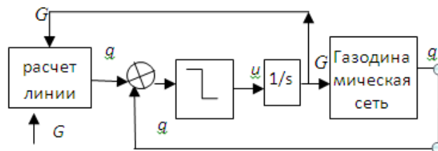
Рисунок 1 – Структура замкнутой системы оптимального по быстродействию управления проветриванием участка
