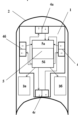
Рисунок 1 – Конструкция модуля системы ориентации АМР
