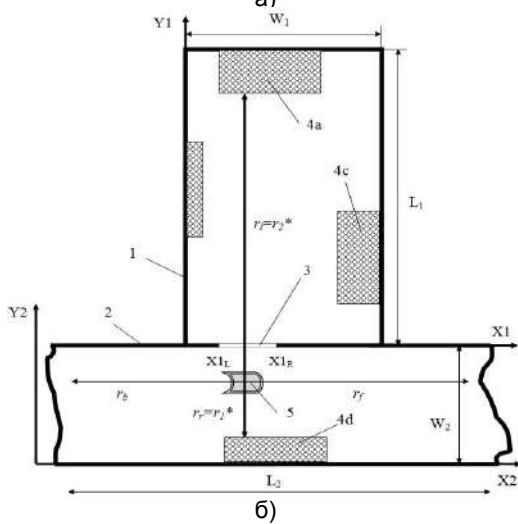
Рисунок 3 – Принцип измерения роботом расстояний до стен в объектно-ориентированной карте помещений: а) в положении робота в начале его движения по комнате 2; б) в положении робота напротив прохода 3 в комнату 1
